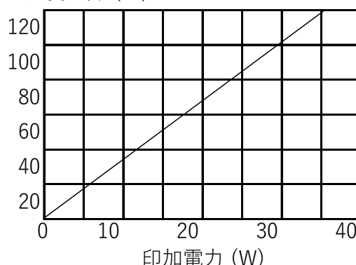
温度上昇 (°C)
